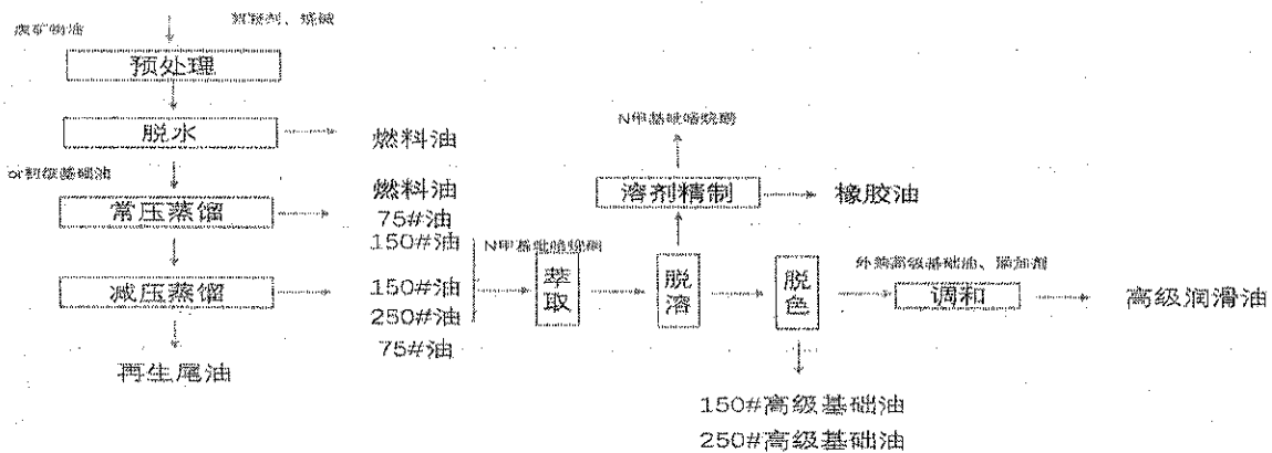
苏州中昊绿能科技有限公司工艺流程图
